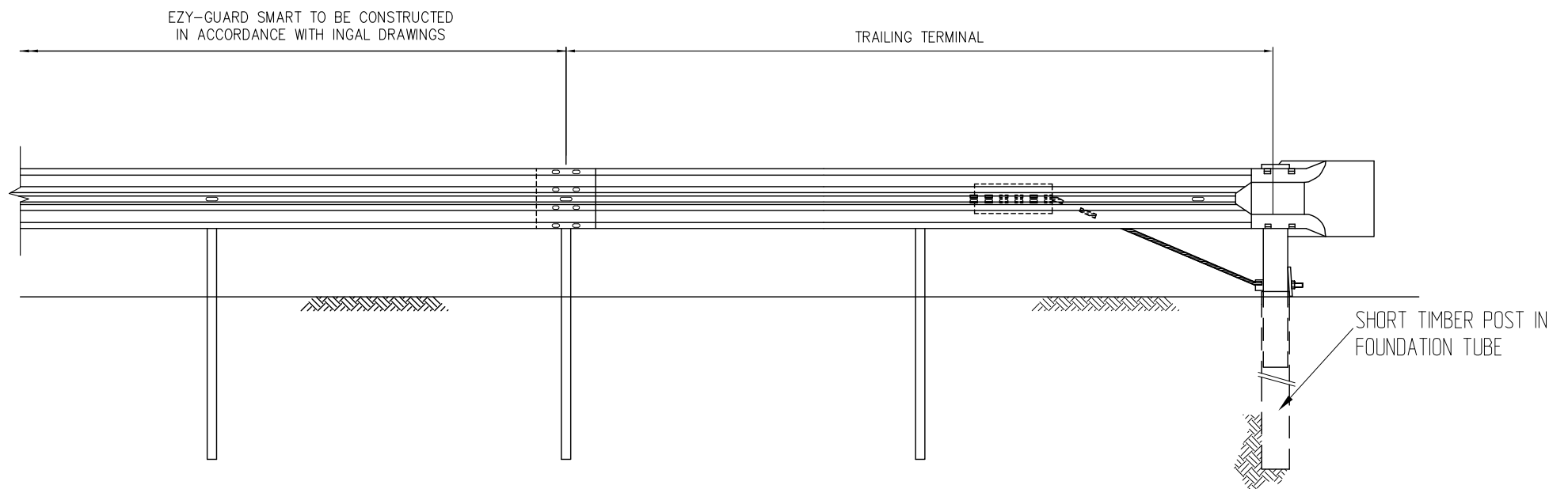
ELEVATION
